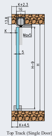
Hi Slide SD 15
