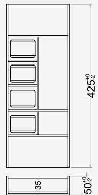
WDO2-WB2
